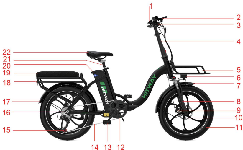
Figura 1 (diagrama de vehículo completo)
