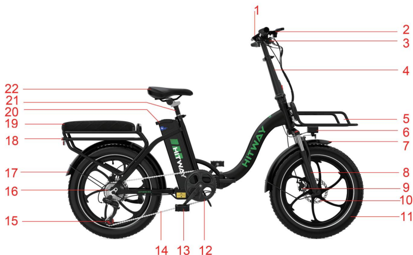
Figura 1 (schema generale del veicolo)
