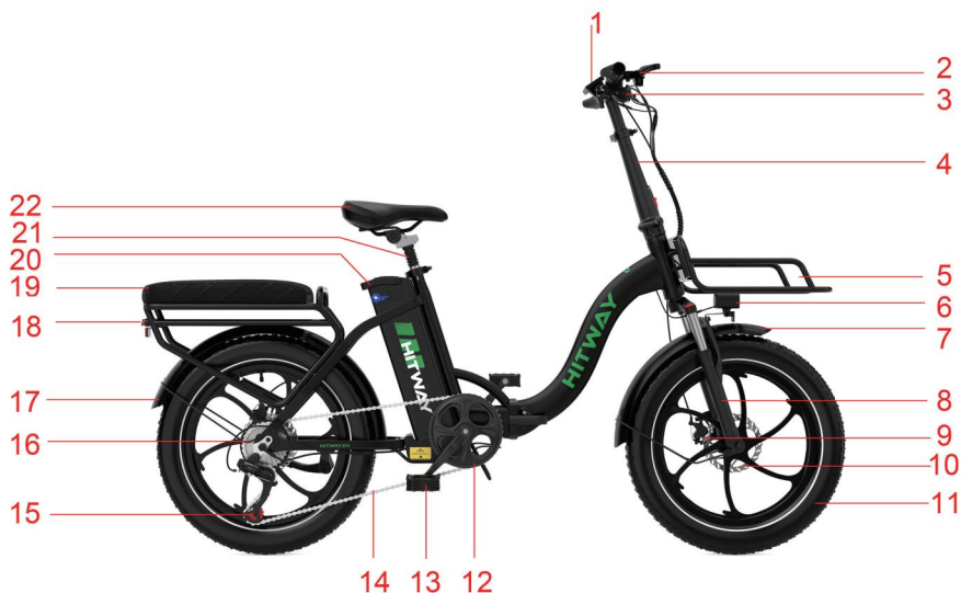
Abbildung 1 (Gesamtfahrzeugdiagramm)
