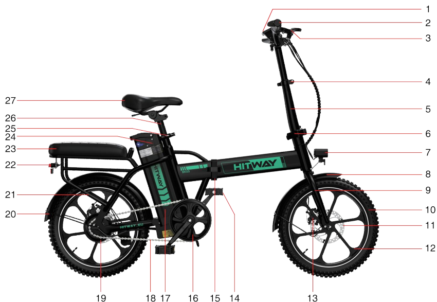
Figure 1 (schéma général du vélo)
